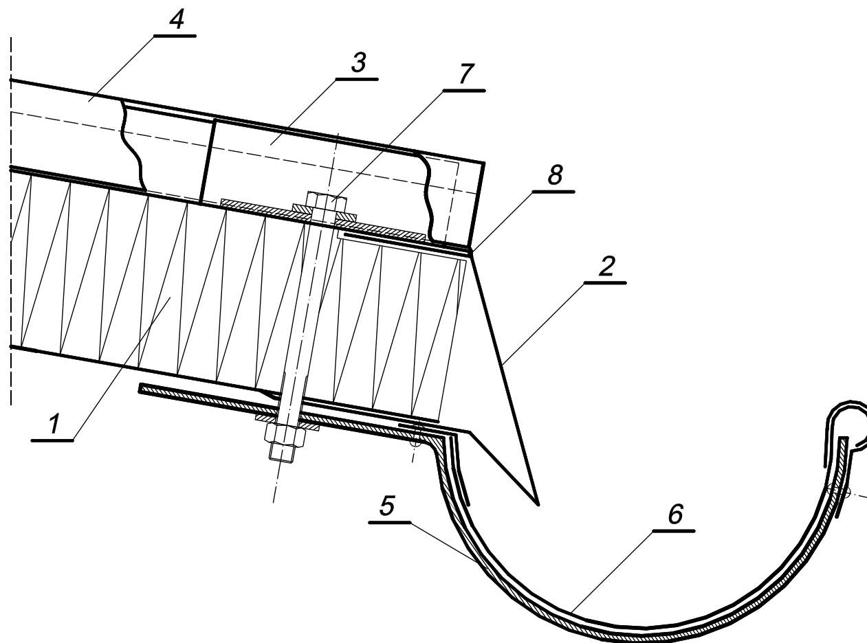
1 - płyta dachowa Prometplast D80 lub D100, 2 - obróbka blacharska OKDZ, 3 - łącznik z blachy ocynkowanej ŁD 4 - obróbka blacharska LD, 5 - hak do rynny, 6 - rynna, 7 - śruba M8 ocynk, 8 - masa uszczelniająca
